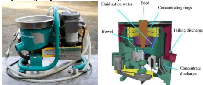
1-rasm. Knelson MD3 markazdan qochirma konsentratiori sxemasi.
