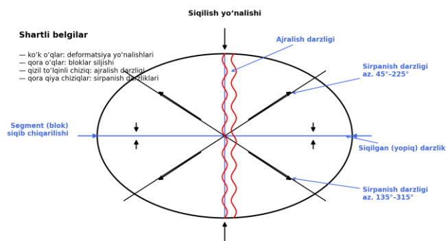
1-rasm. Deformatsiya ellipsoidi va uzilmalar tizimining shakllanishiga oid nazariy sxema.
