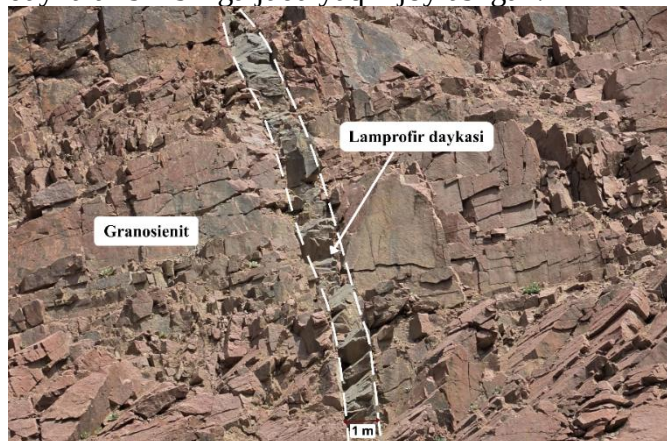
2-rasm. Beshqo'l massivida lamprofir daykalari.
