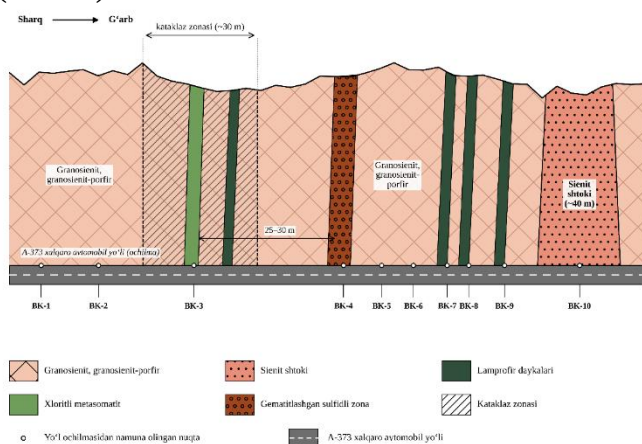
2-rasm. A-3---Beshqo'l kichik intruzivining sxematik kesmasi (BK-1 – BK-10 namunalar olingan tartibda; dala kuzatuvlari asosida, masshtabsiz, tanalarning o'zaro joylashuvi shartli).
