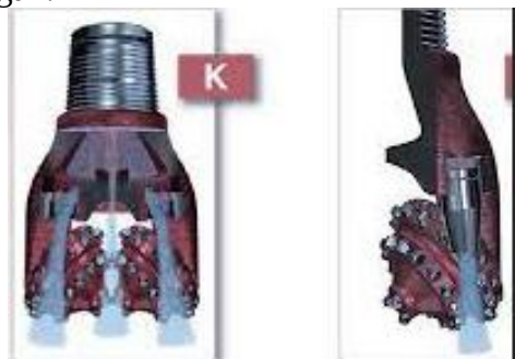
3-rasm. Dolotaning periferik yuvish sxemasi va yuqori tezlikdagi gidromonitor oqimining quduq tubiga ta'siri.
