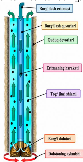
2-rasm. Burg‘ilash qorishmasining dolota orqali quduq tubiga yo‘naltirilishi va shlamning halqa oralig‘i bo‘ylab yer yuzasiga chiqarilishi.
