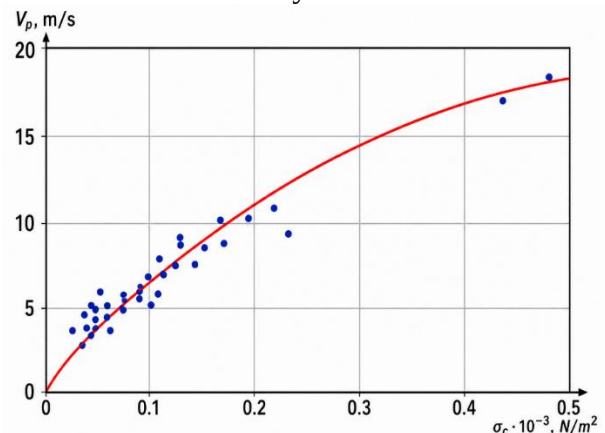
3-rasm. Tajriba kanali qarshiligini hisobga olgan holda chegaraviy (kritik) dinamik tezlikni aniqlash (Mirxulava o'lchovlari bo'yicha).
