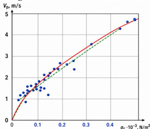
1-rasm. Bog'langan gruntning yuvilish sharti.
