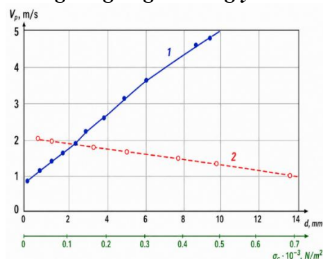
2-rasm. Yopishish va agregat yirikligining kritik tezlikka ta'siri (Mirxulava ma'lumotlari bo'yicha).
