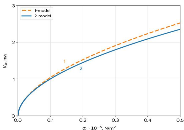
4-rasm. Taqqoslash grafigi: Mirsxulava; - Borovkov.
