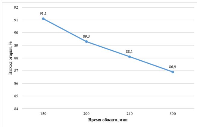
Рис.1. Зависимость выхода огарка от времени обжига руды Сиджакского месторождения Исходное количество ванадия 2400 г/т, T=700 0 С, Расход технической соды Na 2 CO 3 50 г/кг.
