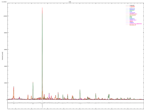
Рис.1. Порошковая дифрактограмма образца.
