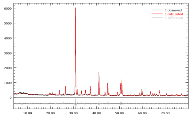
1-rasm. Saponitning rentgenogrammasi.
