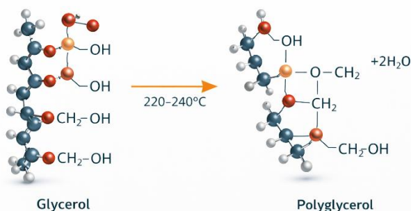
3-rasm. Glitserinning termik degidratatsiyasi natijasida poligliserol hosil bo‘lish reaksiyasi.
