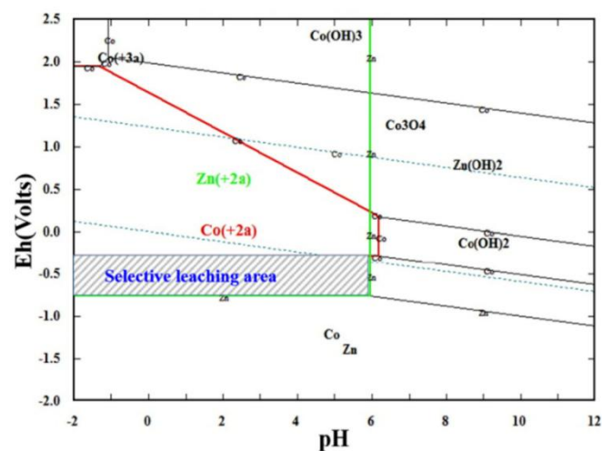
Рис.1. Диаграмма Eh-pH системы Zn-Co-H 2 O при 25 °С.
