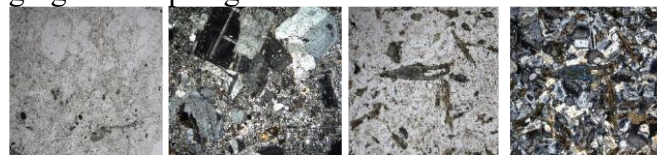
3-rasm. Bokali intruzivining daykali faza jinslari:
