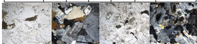
2-rasm. Bokali intruzivining asosiy fazasi jinslari:
