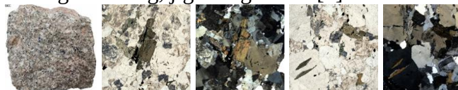
3-rasm. Di-70 adamelitning petrografik ko'rinishlari:
