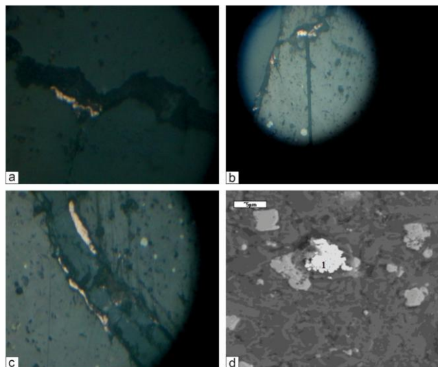
3-rasm. Sof tug'ma oltin va kumushning ajralish shakllari:
