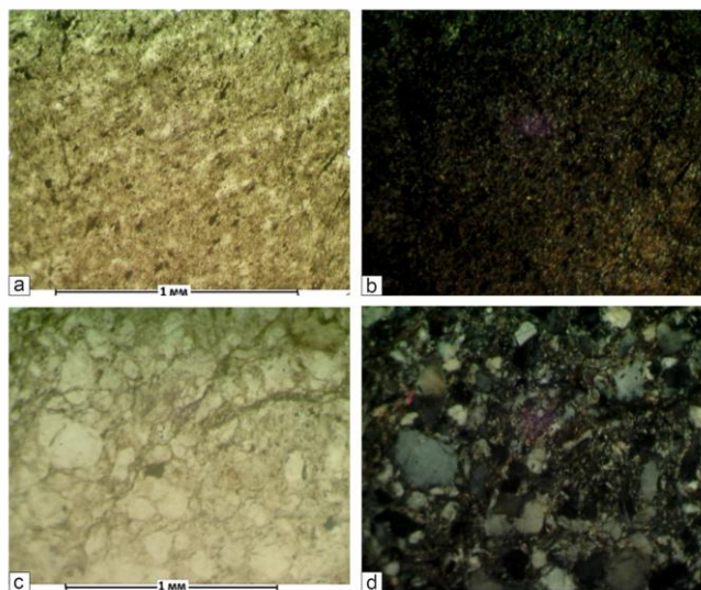
1-rasm. Tufogen metaalevrolit va metaquartzitlarning mikrostrukturaviy xususiyatlari:
