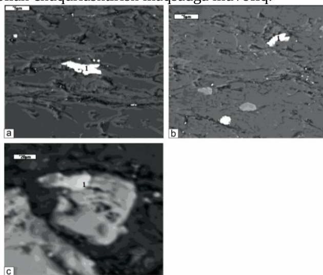
5-rasm. Neodimli monatsit va ksenotim ajralmalarining tarkibiy-morfologik xususiyatlari:
