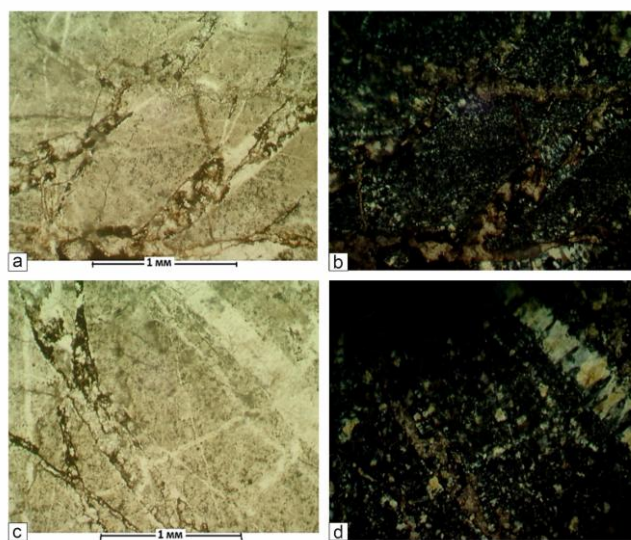
2-rasm. Brekchiyalangan metaalevrolitlardagi tomirli hosilalar:
