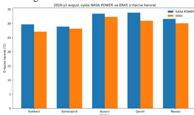
2-rasm. Oʻzbekistonning beshta shahrida NASA POWER va ERA5 maʼlumotlari boʻyicha oʻrtacha havo haroratining taqqoslanishi.
