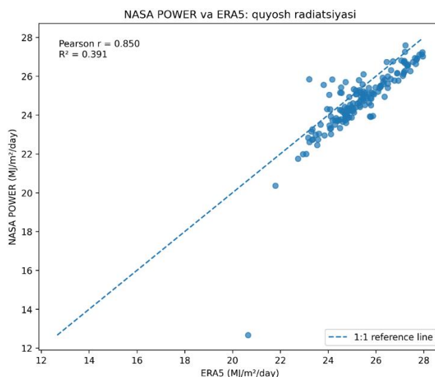
5A-rasm. Quyosh radiatsiyasi.
