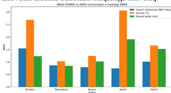
4-rasm. NASA POWER va ERA5 ma'lumotlari o'rtasidagi RMSE qiymatlarining hududlar bo'yicha taqqoslanishi.
