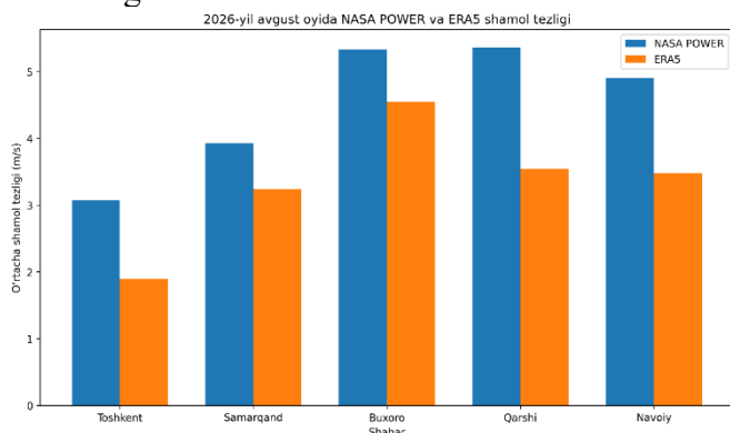
3-rasm. O'zbekistonning beshta shahrida NASA POWER va ERA5 ma'lumotlari bo'yicha o'rtacha shamol tezligining taqqoslanishi.
