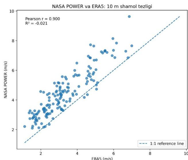
5C-rasm. Shamol tezligi.
