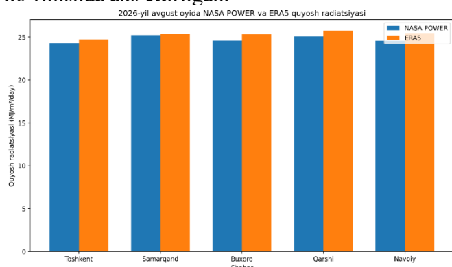
1-rasm. Oʻzbekistonning beshta shahrida NASA POWER va ERA5 maʼlumotlari boʻyicha oʻrtacha kunlik quyosh radiatsiyasining taqqoslanishi.
