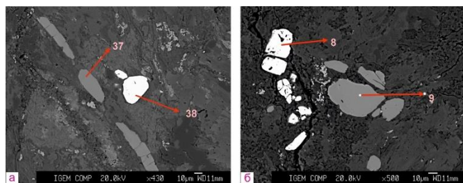
Рис.7. Морфология выделений апатита (а, б) и пирита.
