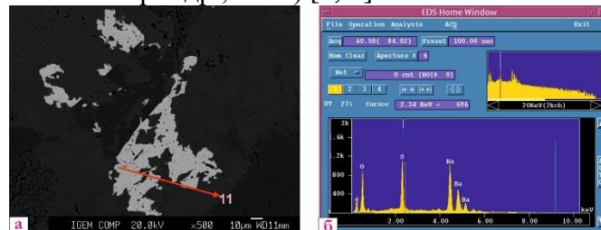
Рис.6. Морфология выделений барита.
