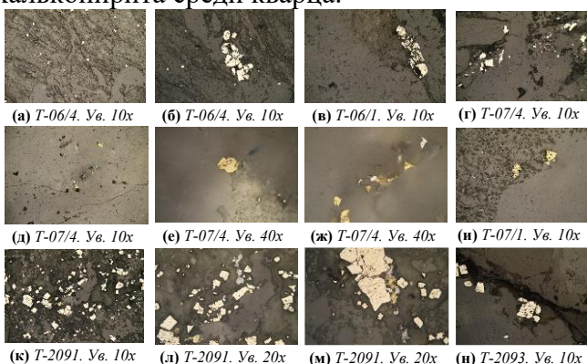
Рис.2. Характер распределения и морфология выделений пирита и других рудных минералов. Проявление Самарчук. Микрофото в отраженном свете.
