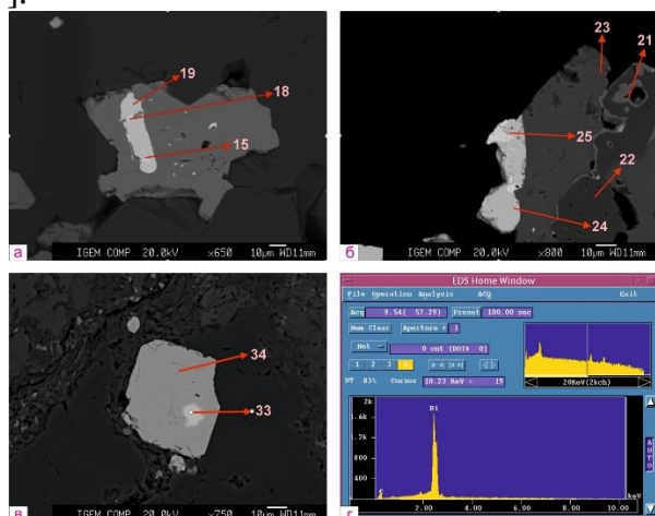
Рис.5. Взаимоотношения галенита.
