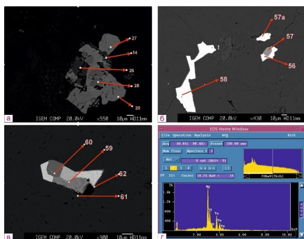
Рис.4. Сросток халькопирита и пирита с микровключениями апатита.
