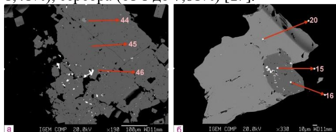
Рис.3. Взаимоотношения рудных минералов в проявлении Самарчук.
