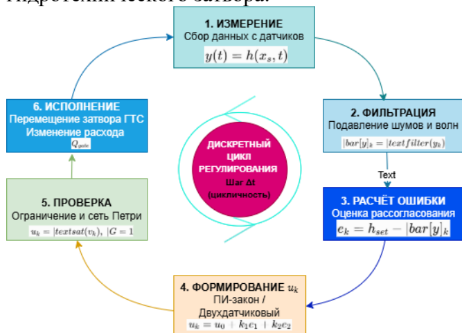
Рис.1. Структура замкнутого алгоритмического цикла регулирования уровня: от метрологической фильтрации измерений до логической верификации и исполнения команды на затворе ГТС.
