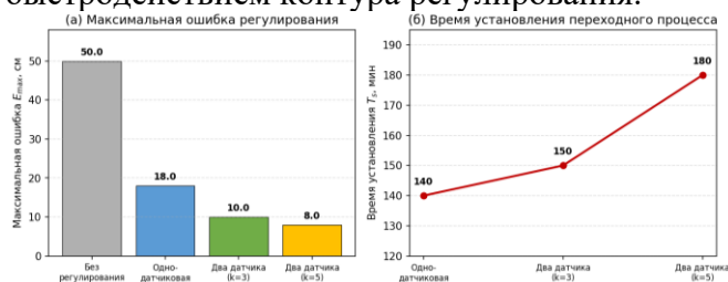
Рис.2. Сравнение максимальной ошибки регулирования E_{\max} (а) и времени установления T_s (б) для различных схем управления по данным таблицы 1.
