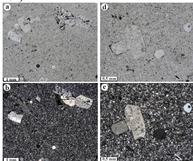
2-rasm. Kvarsli andezit.
