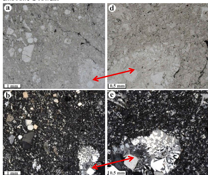
3-rasm. Andezidatsit.
