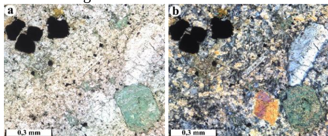
1-rasm. Andezibazaltning petrografik xususiyatlari.
