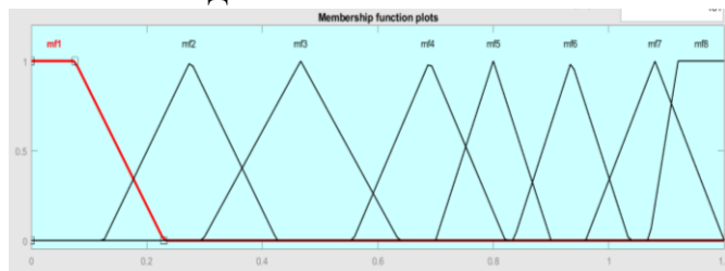
4-расм. Сув омбори тизимидан сув оқиб чиқиши ( m^3/соат ) учун тегишлилик функцияси.
