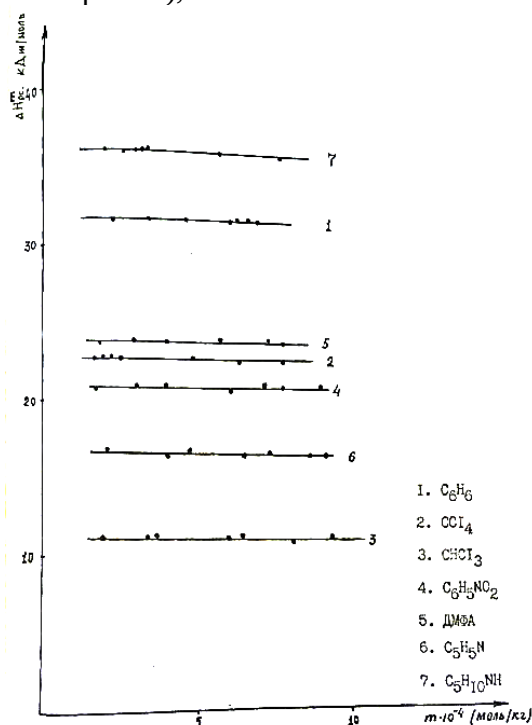
2-rasm. Organik erituvchilarda eritilganda entalpiyaning ( H merish) o'zgarishining H_2Xl(a) konsentratsiyasiga ( 10^{-4} mol/kg) bog'liqligi.
