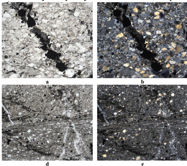
1-rasm. a-b-metamorflashgan tufalevrolit 40 x , d-e- Tufalevrolit bo'yicha rivojlangan kvars-sideritsitli slanes 20 x .
