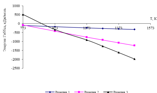
Рис.1. Изменение энергии Гиббса основных реакций образования свинца в зависимости от температуры.
