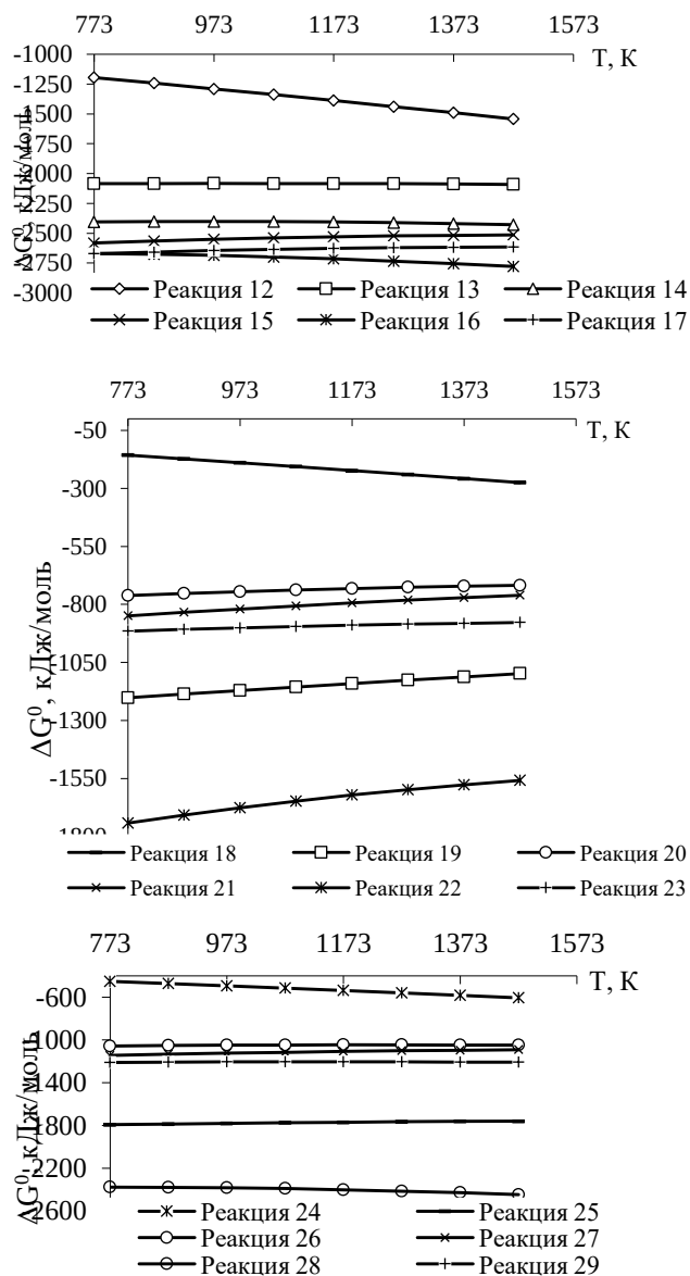
Рис.5. Изменение энергии Гиббса основных реакций возгонки оксидов и сульфидов рения в зависимости от температуры.
