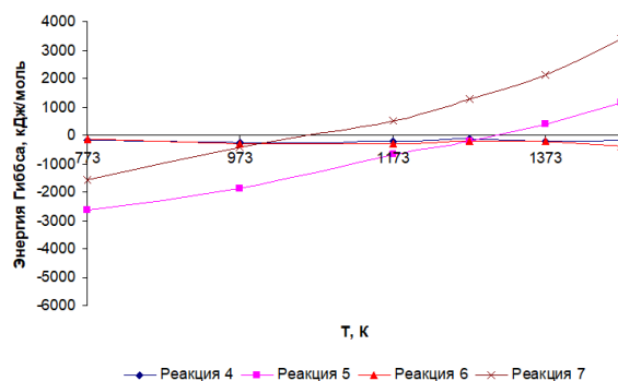
Рис.2. Изменение энергии Гиббса основных реакций концентрации золота, серебра в сплаве со свинцом и образование окситиосолей теллура, селена в зависимости от температуры.
