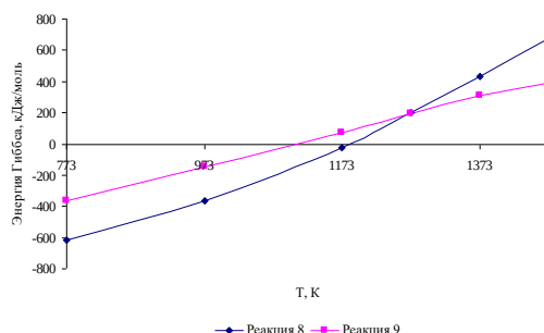
Рис.3. Изменение энергии Гиббса основных реакций разрушения селенатов меди в зависимости от температуры.
