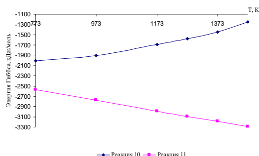
Рис.4. Изменение энергии Гиббса основных реакций разрушения селенидов, теллуридов золота и серебра с образованием тиосолей селена и теллура в зависимости от температуры.
