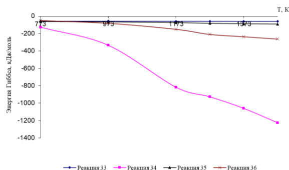
Рис.6. Изменение энергии Гиббса основных реакций образования тиосолей меди и цинка в зависимости от температуры.
