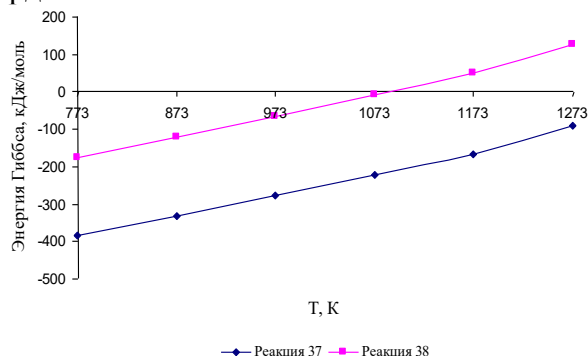
Рис.7. Изменение энергии Гиббса основных реакций образования тиосолей селена и теллура в зависимости от температуры.
