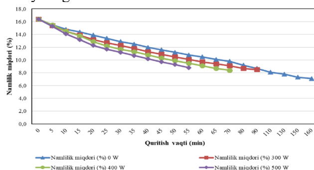
4-rasm. Turli mikroto'liqin quvvatlarida material namligining quritish vaqtiga bog'liqligi. (Manba: Taheri va boshqalar).
