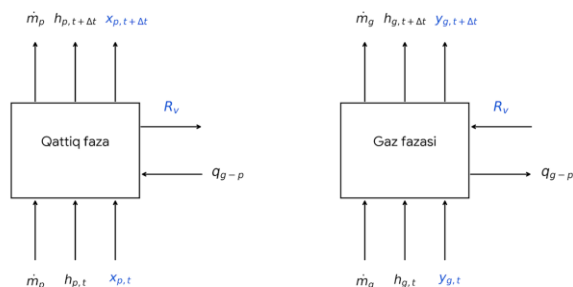
1-rasm. Mavhum qaynash qatlamli quritish jarayonining gaz va qattiq fazalar uchun matematik modeli sxemasi.
