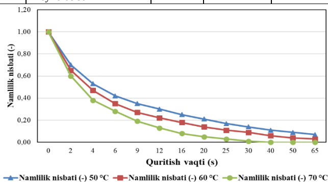
2-rasm. Quritish harorati va namlik nisbatining quritish vaqtiga bog'liqligi. (Manba: Sozzi va boshqalar).
