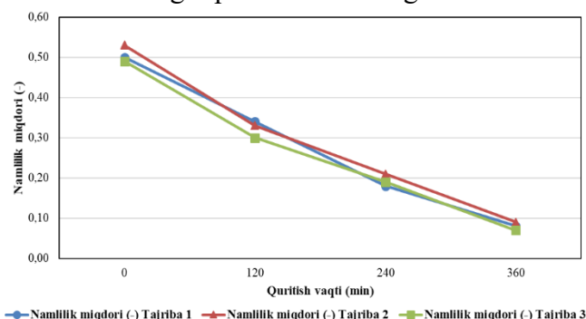
3-rasm. Turli tajriba sharoitlarida namlik miqdorining quritish vaqtiga bog'liqligi. (Manba: Mohseni va boshqalar).
