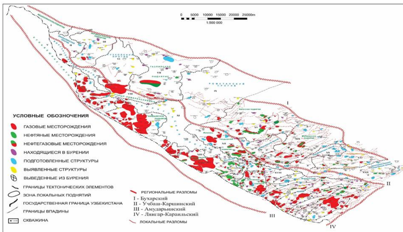
Рис.1. Схематическая тектоническая карта Бухаро-Хивинского региона с размещением месторождений нефти и газа и перспективных площадей.
