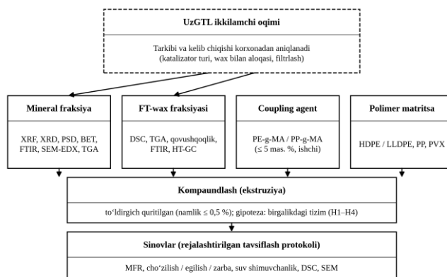
2-rasm. UzGTL mineral fraksiyasi, FT-wax va coupling agentning birgalikdagi tizimi (taklif etilgan sxema).
