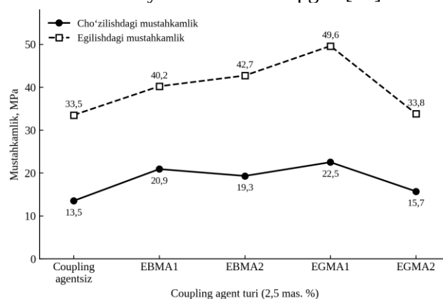
1-rasm. HDPE/RH kompozitlarining mustahkamligi (Arjmandi [2] sharhidagi 6-jadval ma'lumotlari asosida chiziqli grafik shaklida qayta chizilgan).
