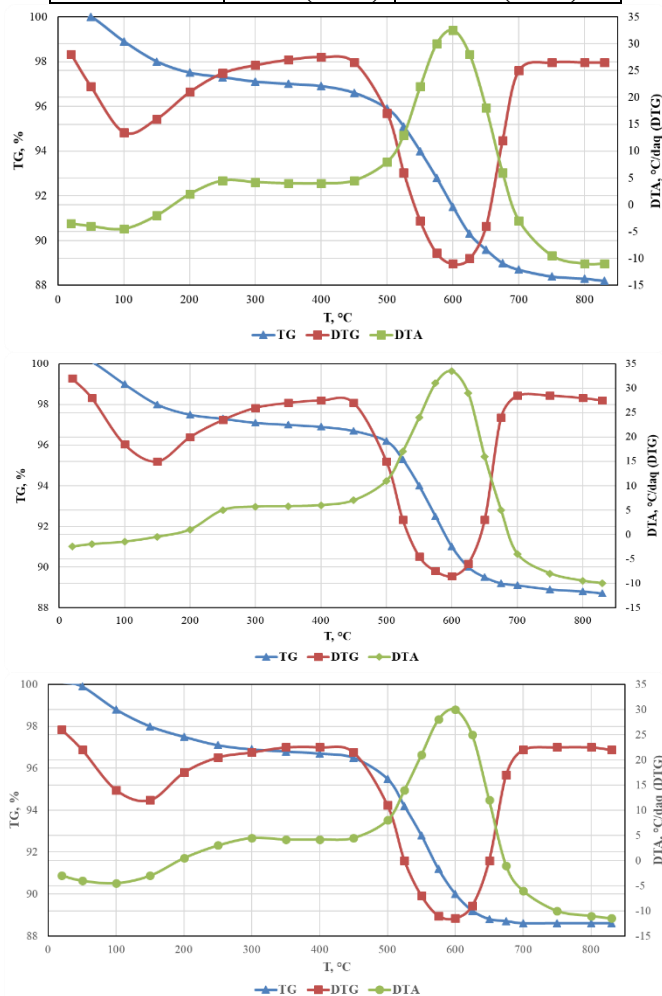
1-rasm. Rux aluminosilikatlarining propan bilan 6 soat davomida ishlov berilgandan keyingi termogrammalari.
