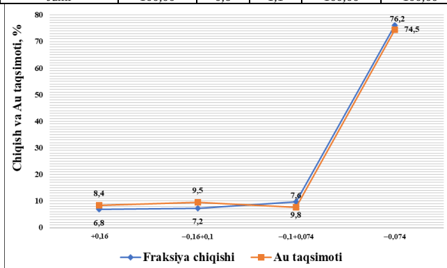
1-rasm. GMZ-3 texnogen chiqindilarida fraksiyalar massa chiqishi va oltin taqsimoti (muallif ishlanmasi).
