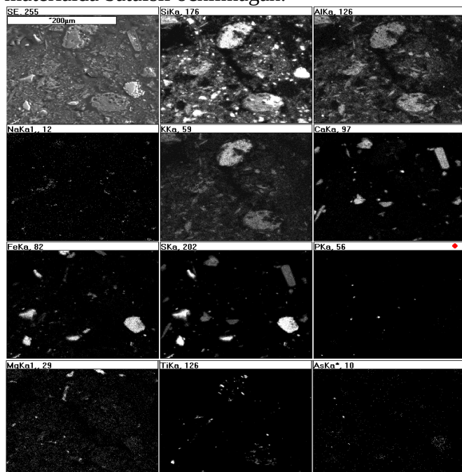
2-rasm. GMZ-3 chiqindilarining 8-namunasidagi elektron tasvir va Si, Al, Na, K, Ca, Fe, S, P, Mg, Ti hamda As elementlari tarqalish xaritalari (muallif ishlanmasi).
