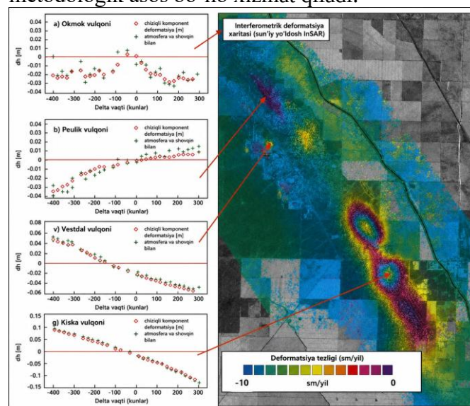
3-rasm. Boshlang'ich hujjatda Lost Hills deb berilgan kompozit.
