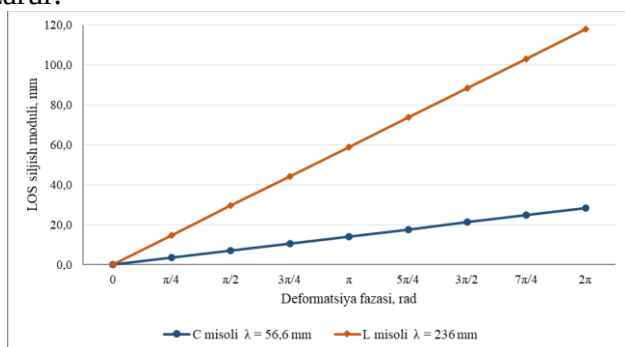
6-rasm. Faza va LOS siljishi orasidagi hisobiy bogʻlanish (Muallif ishlanmasi).
