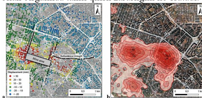
1-rasm. Berezniki hududidagi deformatsiya maydonining nuqtaviy (a) va izoliniyal (b) ko'rinishlari.
