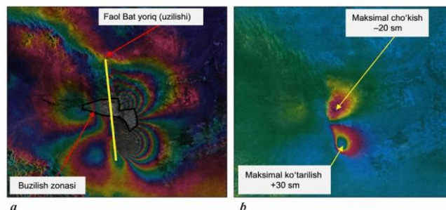
2-rasm. Bam hududiga oid interferometrik kompozit.
