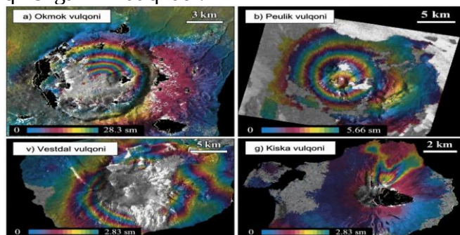
5-rasm. Okmok, Peulik, Westdahl va Kiska vulqonlariga oid interferometrik tasvirlar.
